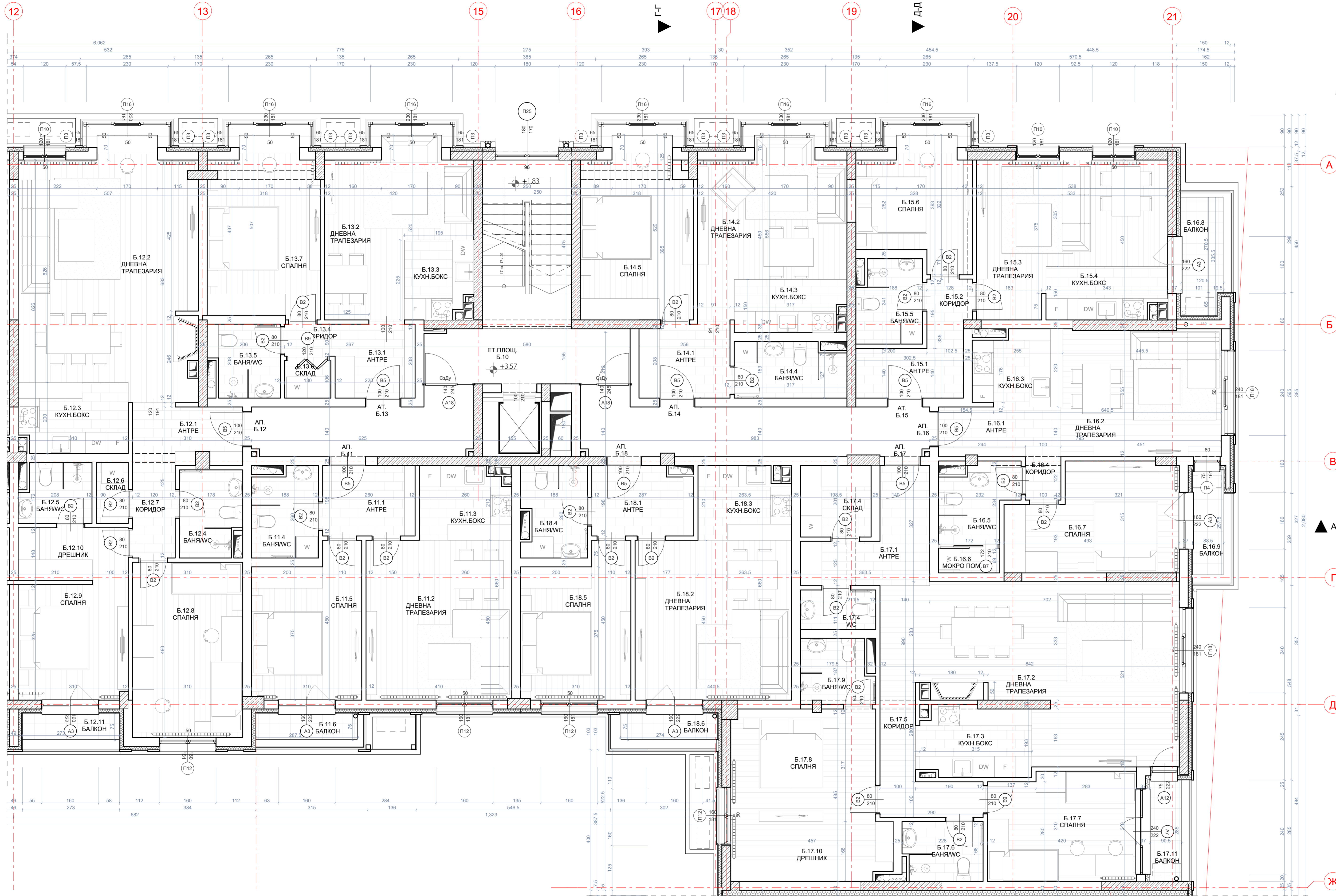
СЕКЦИЯ Б - ЕТАЖ 1 КОТА +3.57
