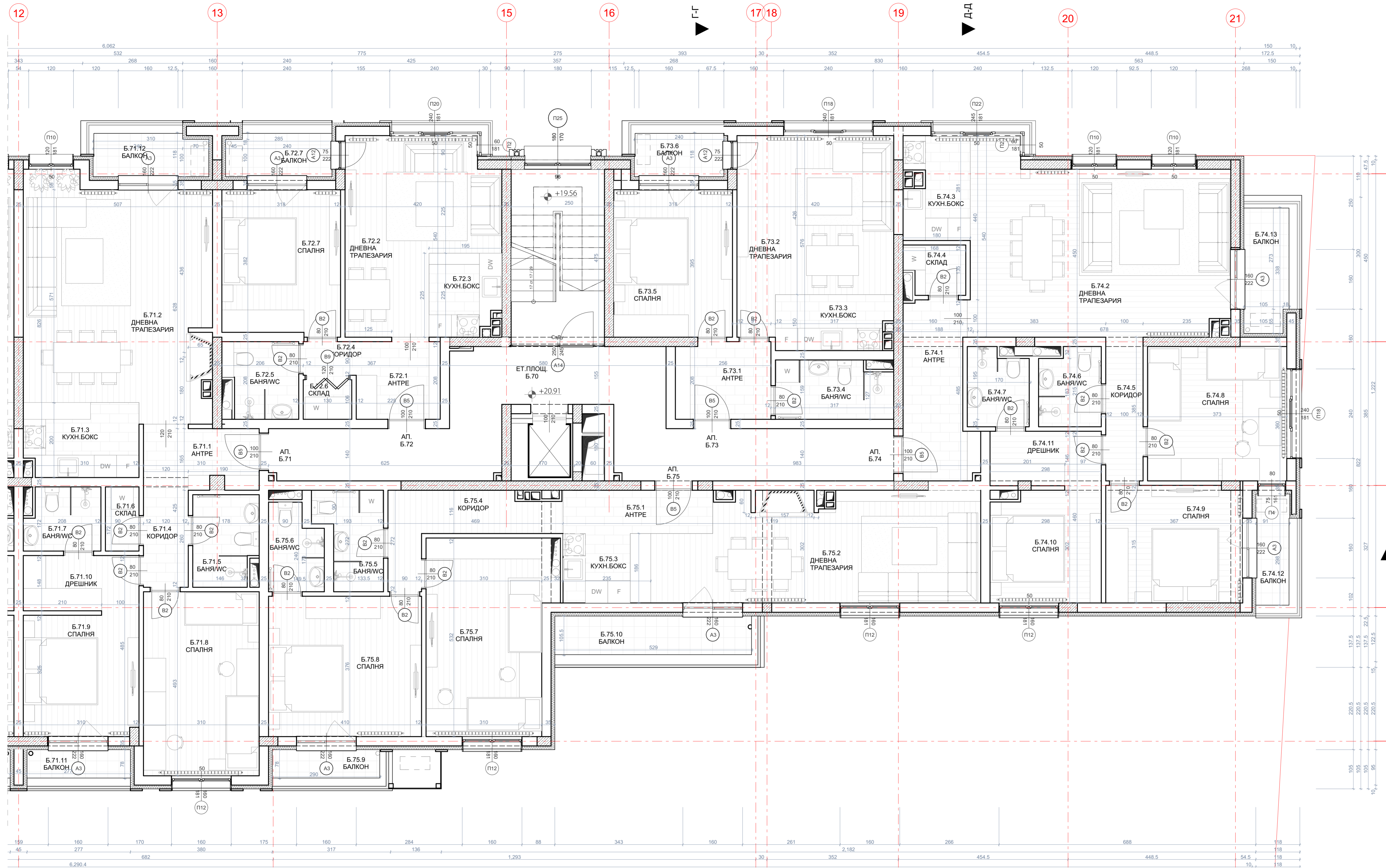
СЕКЦИЯ Б - ЕТАЖ 7 КОТА +20.91
