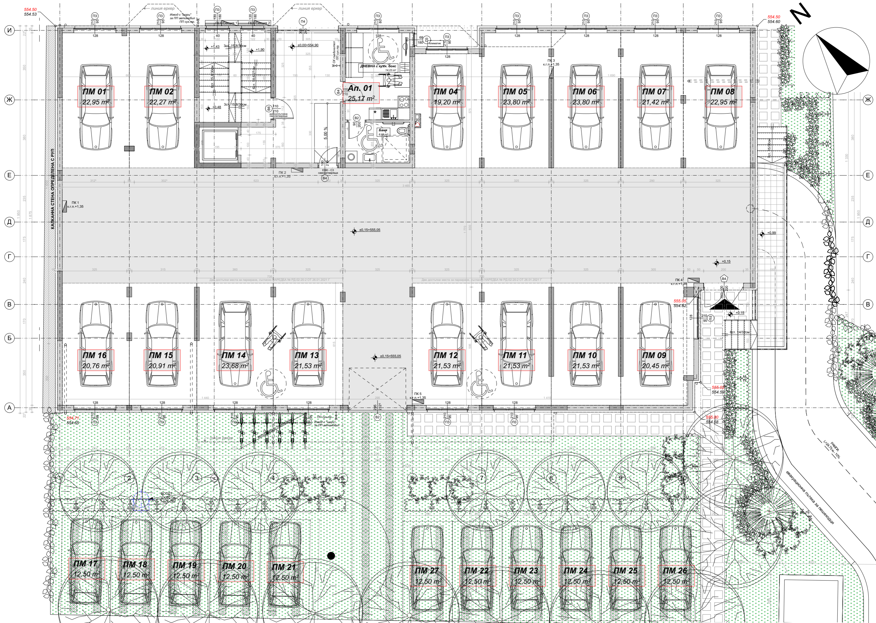
РАЗПРЕДЕЛЕНИЕ ПАРТЕР
