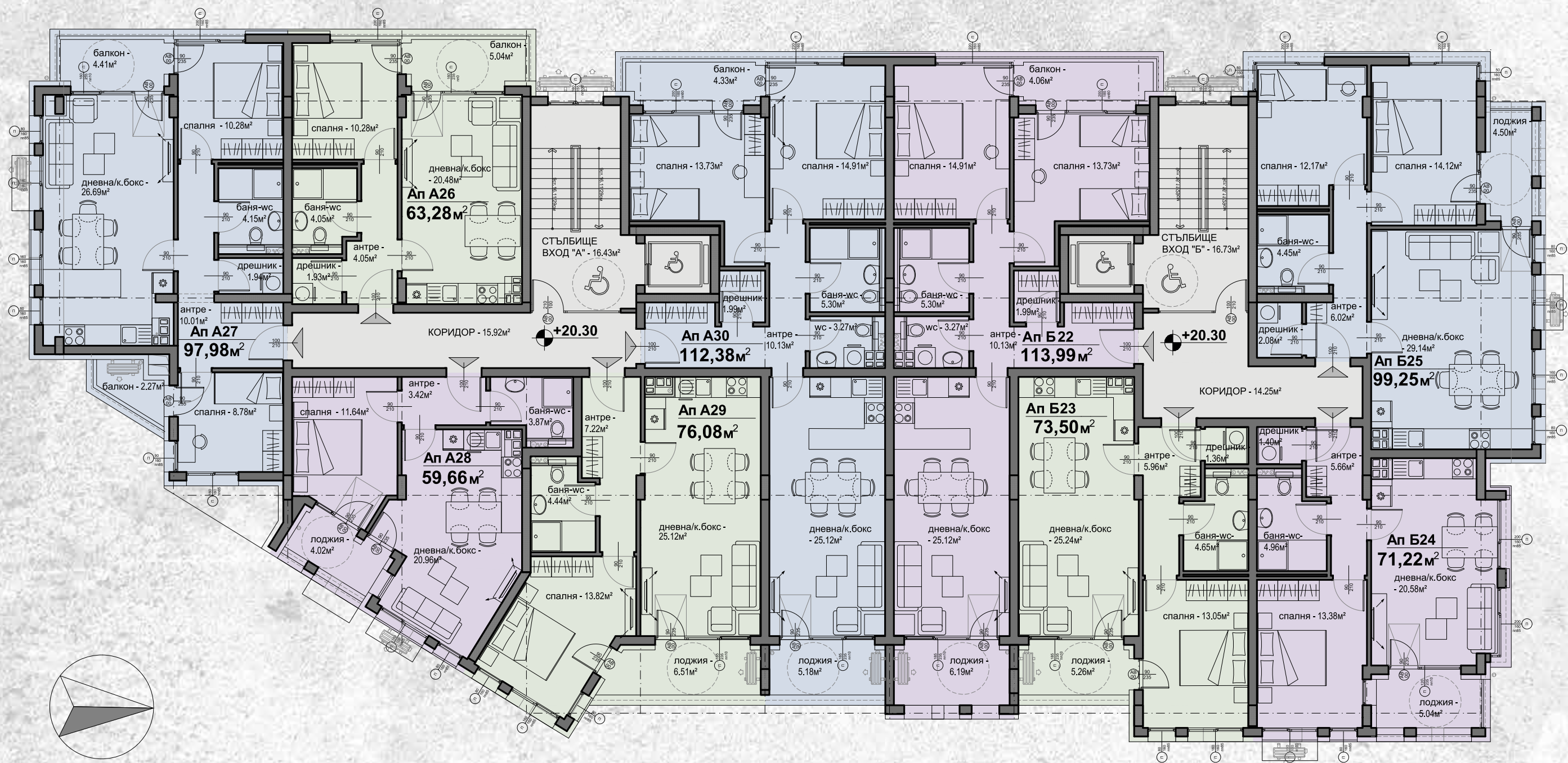
РАЗПРЕДЕЛЕНИЕ ШЕСТИ ЕТАЖ, М 1:150
