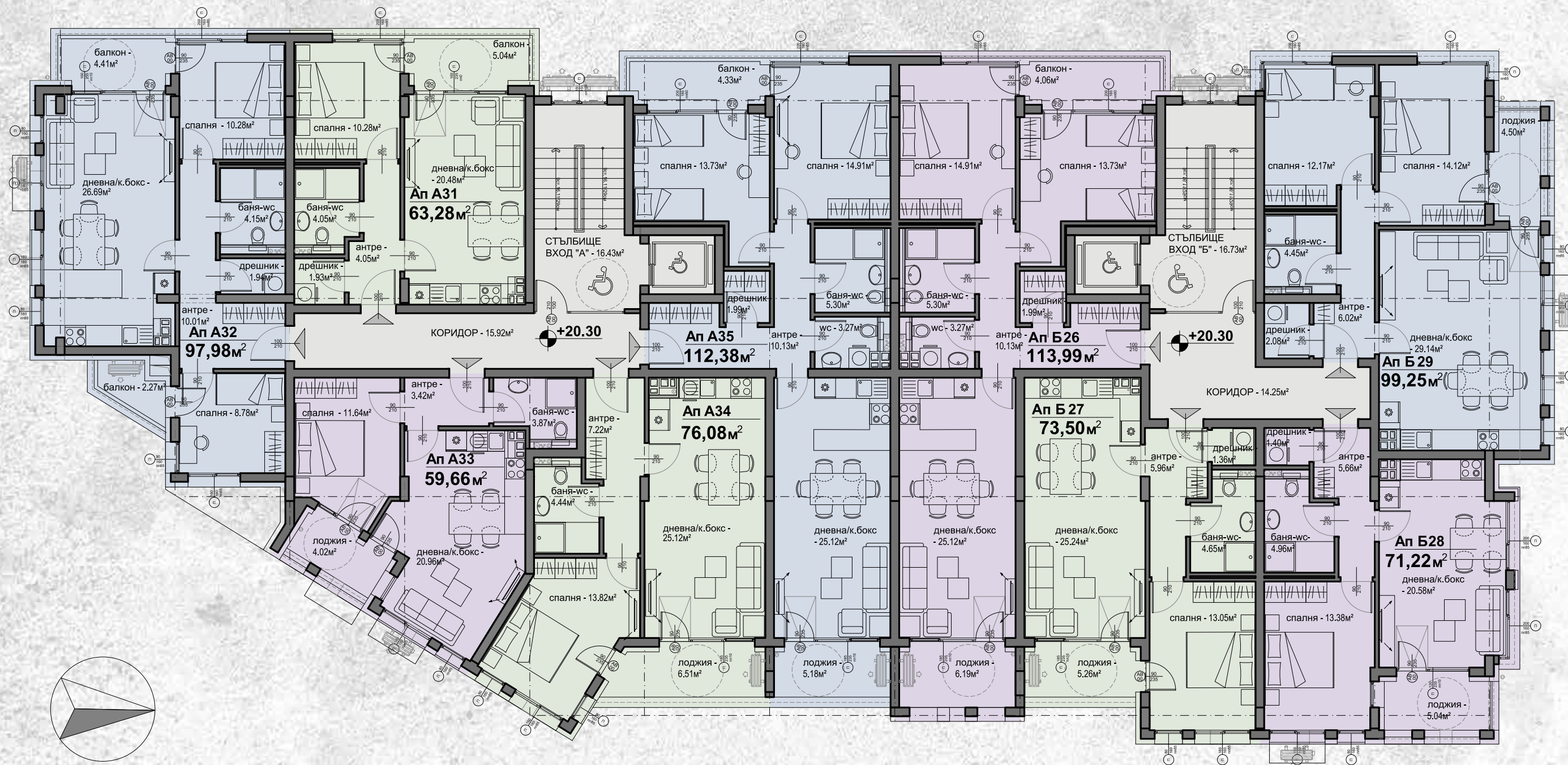
РАЗПРЕДЕЛЕНИЕ СЕДМИ ЕТАЖ, М 1:150
