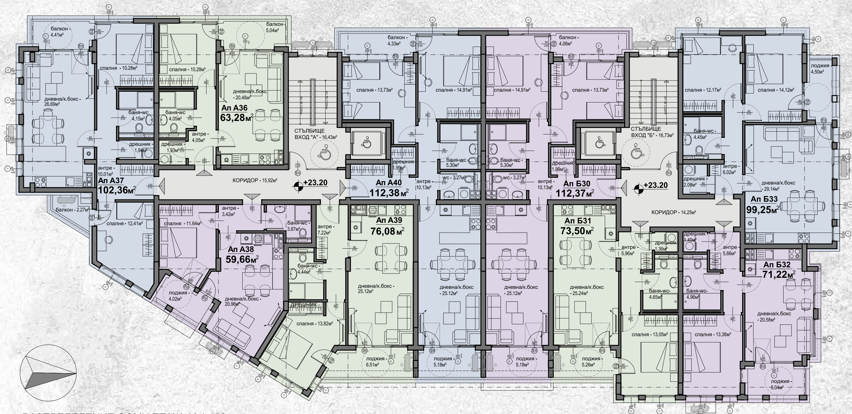
РАЗПРЕДЕЛЕНИЕ ОСМИ ЕТАЖ, М 1:150
