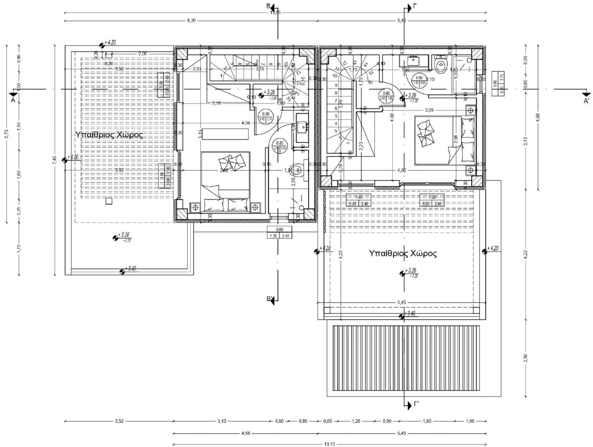
ΚΑΤΟΨΕΙΣ ΣΟΦΙΤΩΝ
