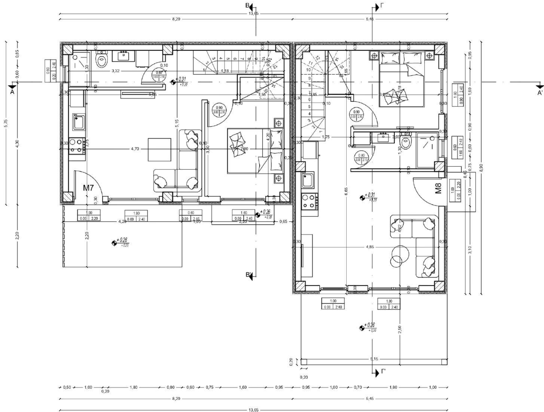
ΚΑΤΟΨΕΙΣ ΙΣΟΓΕΙΟΥ
