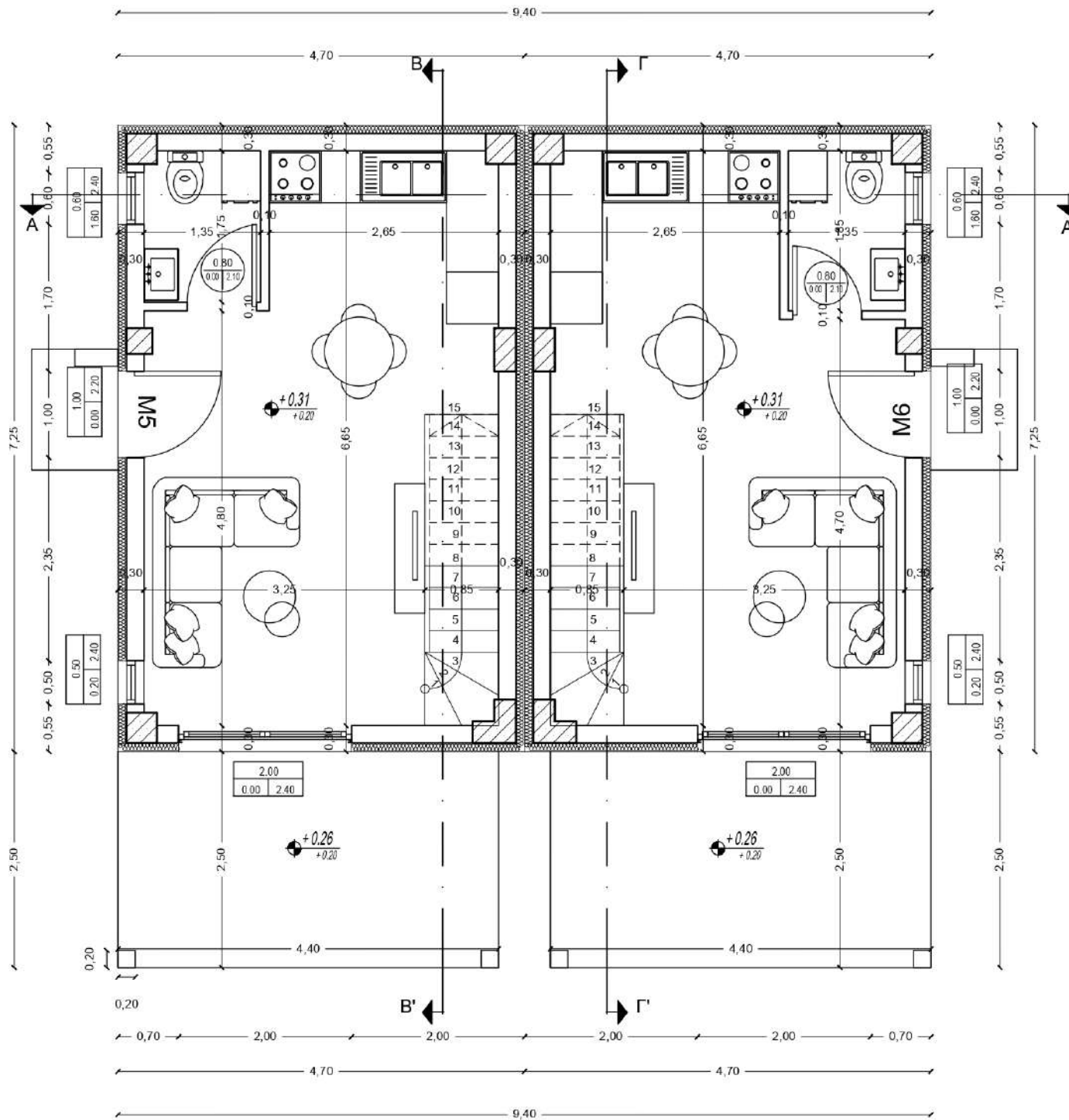
ΚΑΤΟΨΕΙΣ ΙΣΟΓΕΙΟΥ
