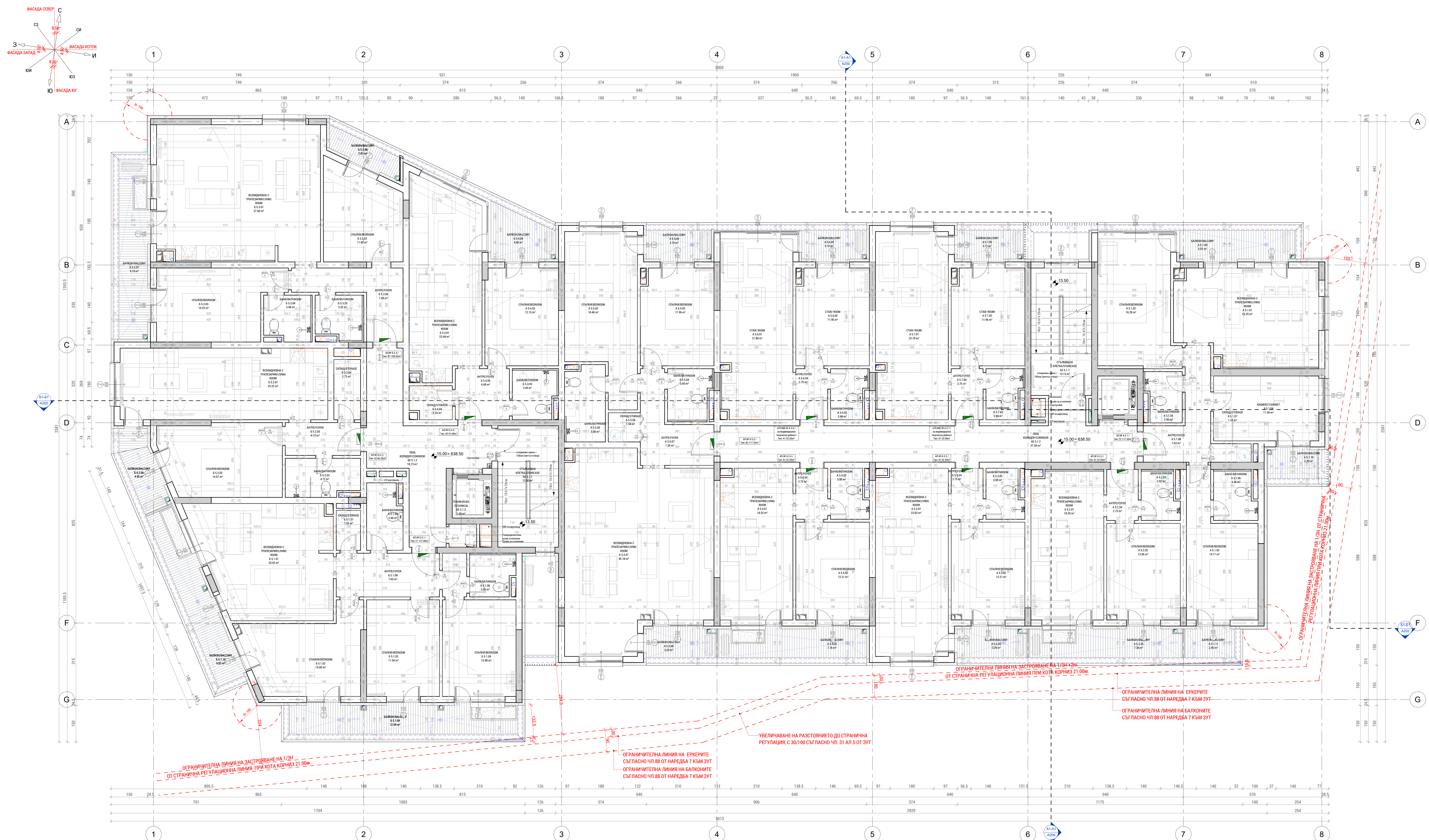
ЗАСТРОЕНА ПЛОЩ ПЕТИ ЕТАЖ - 959.78m 2
