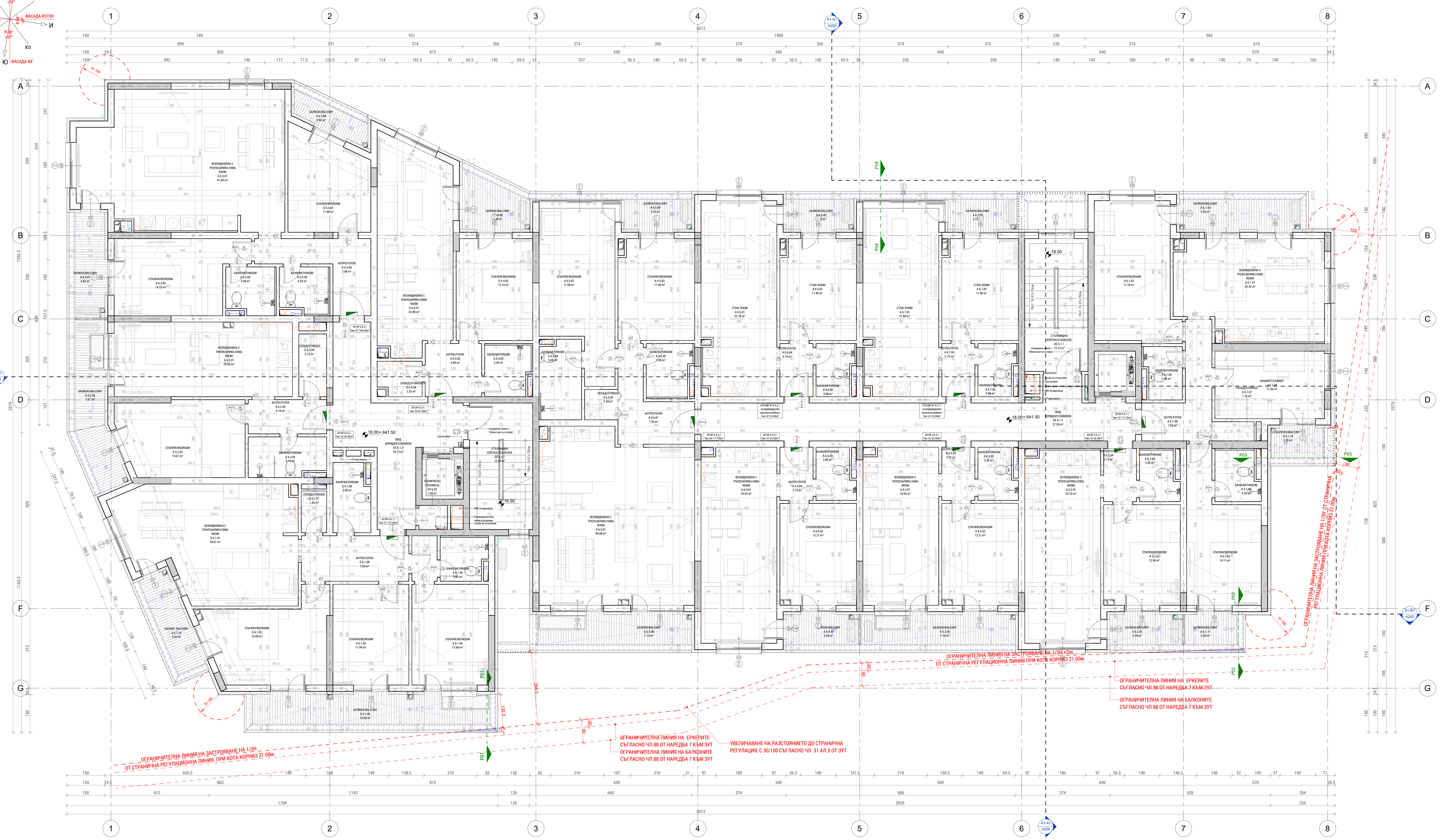
ЗАСТРОЕНА ПЛОЩ ШЕСТИ ЕТАЖ - 959.78m 2
