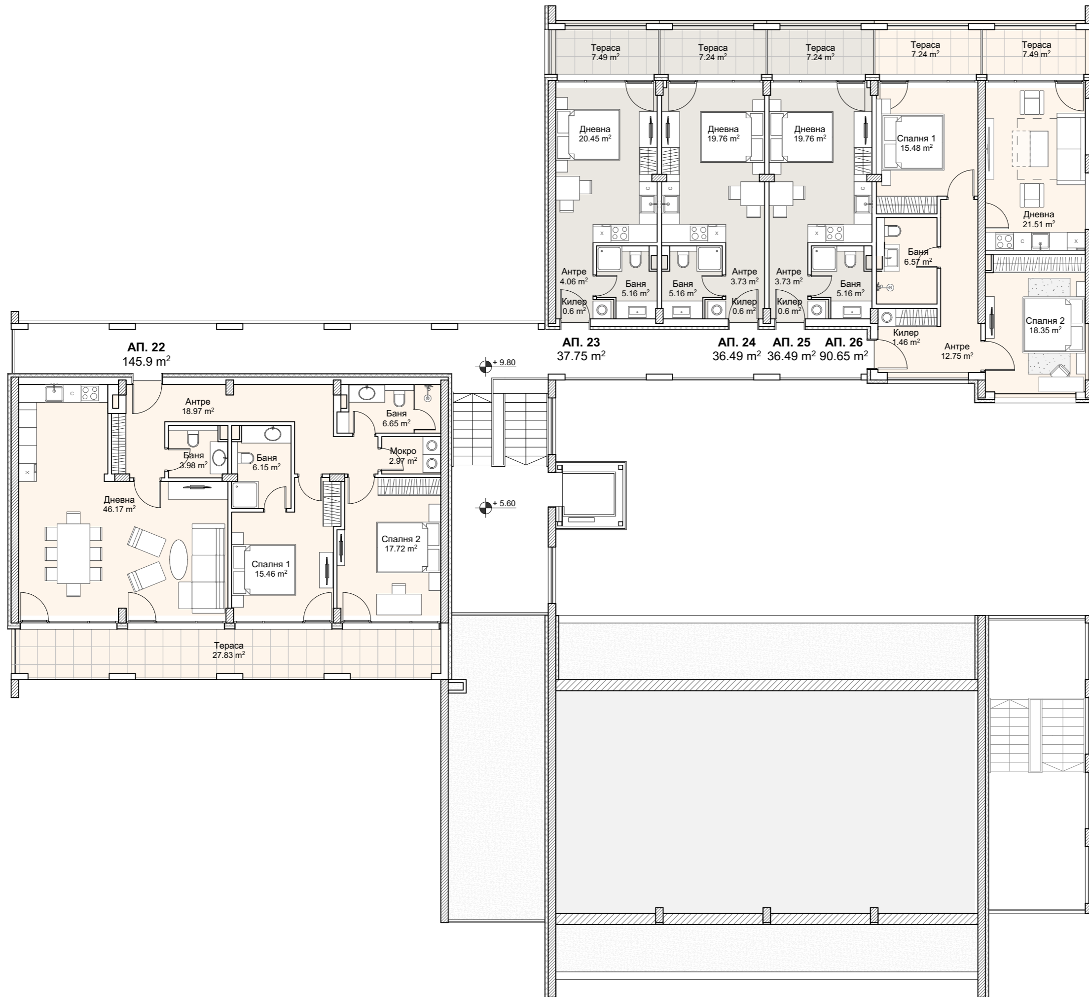
БЛОК 3 ПЛАН НА КОТА +9.80
