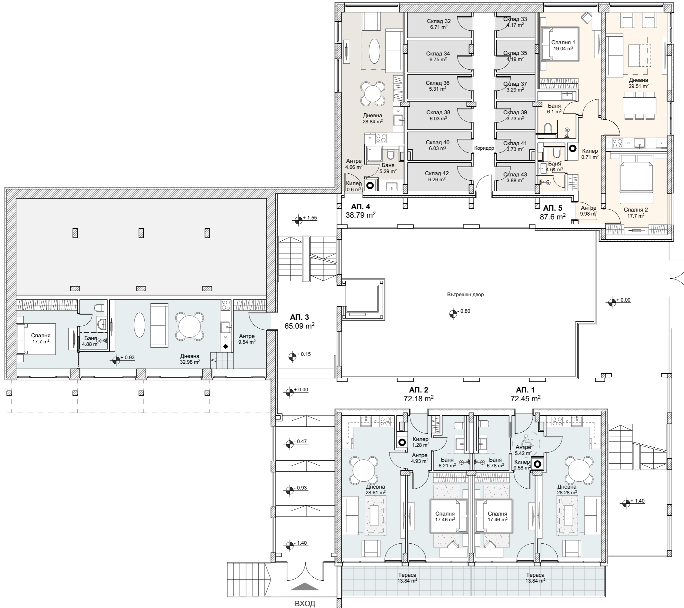
БЛОК 3 ПЛАН НА КОТА +0.00/+1.40
