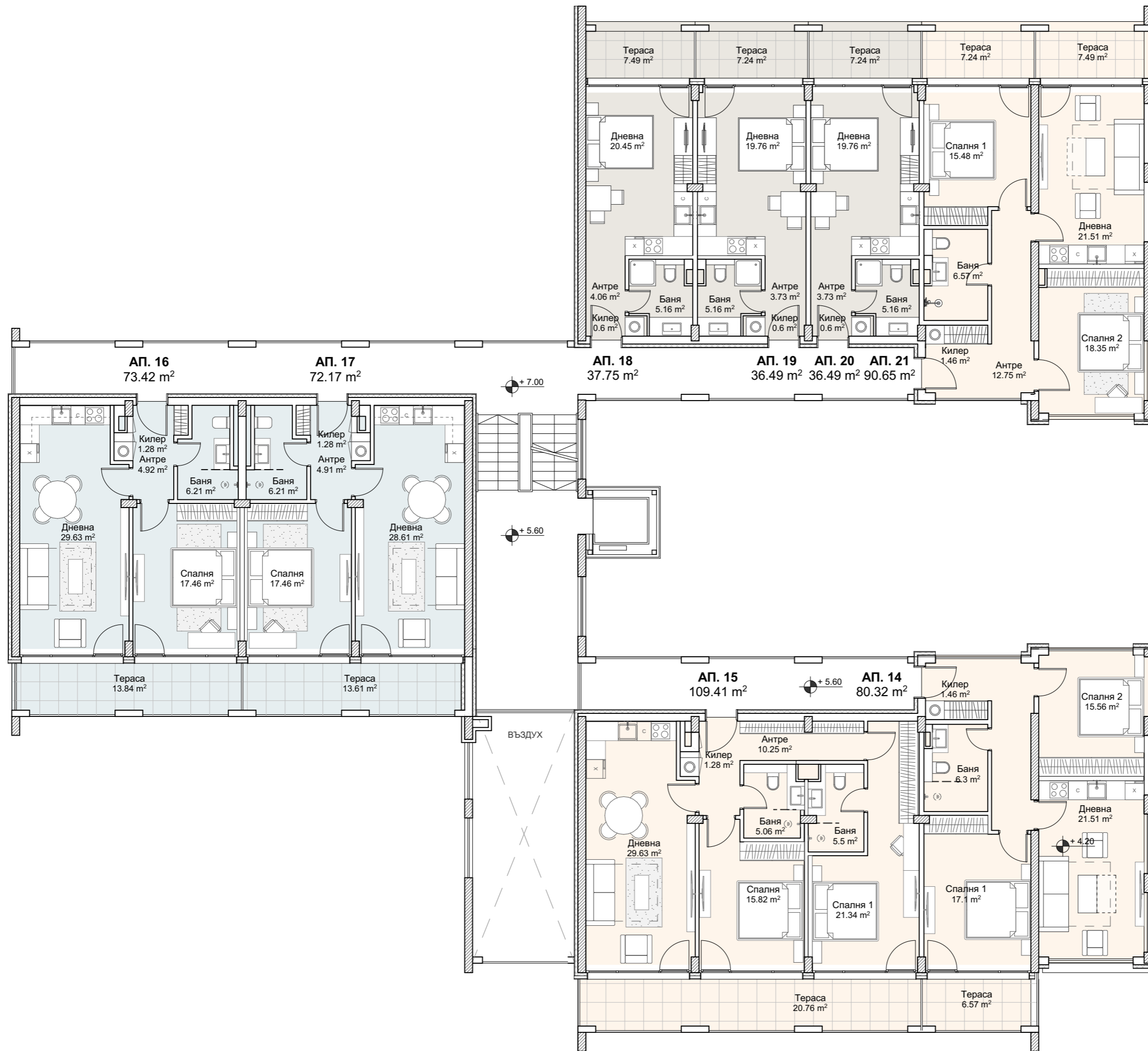
БЛОК 3 ПЛАН НА КОТА +5.60/+7.00
