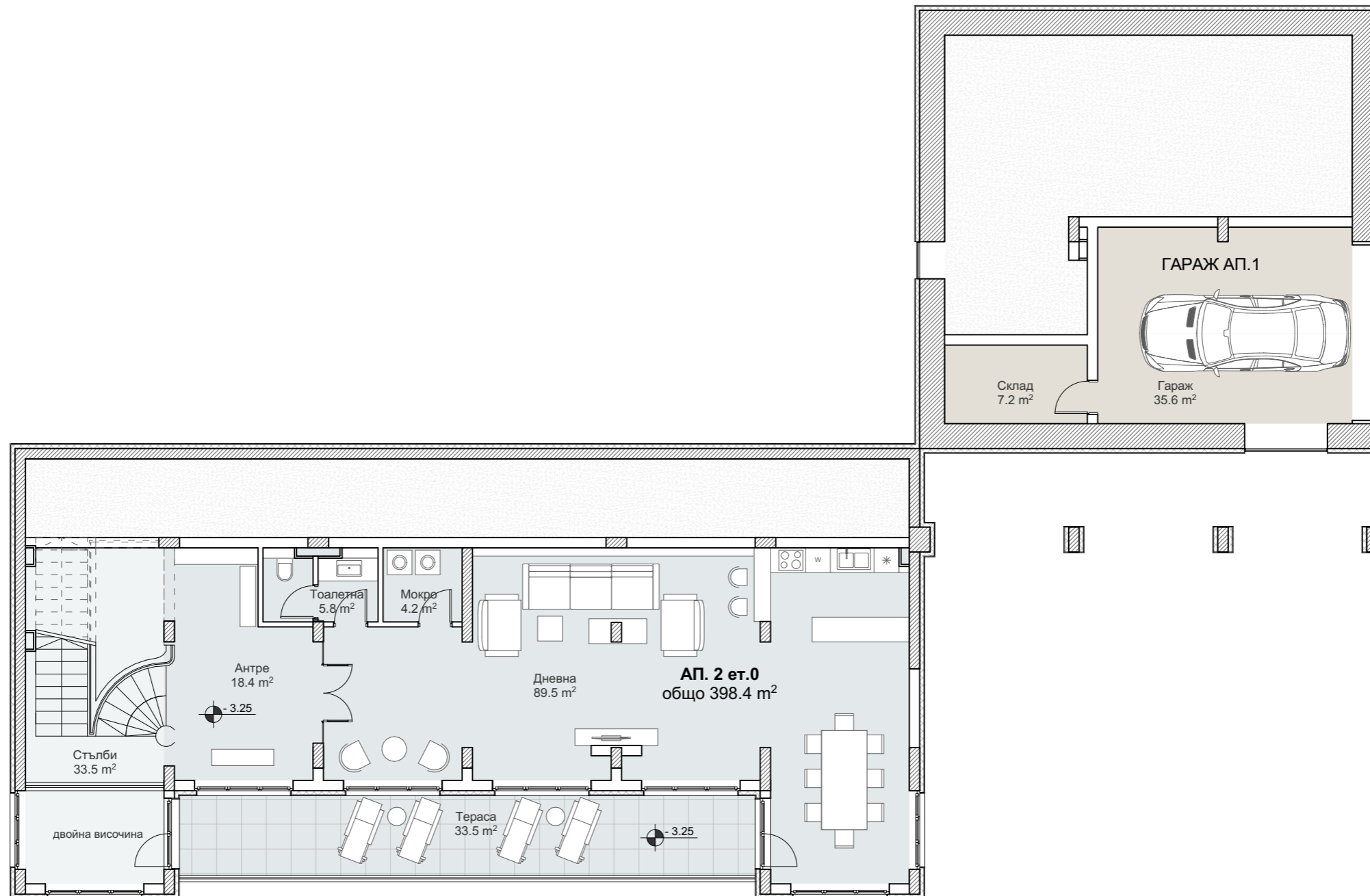
БЛОК 2 ПЛАН НА КОТА - 3.25
