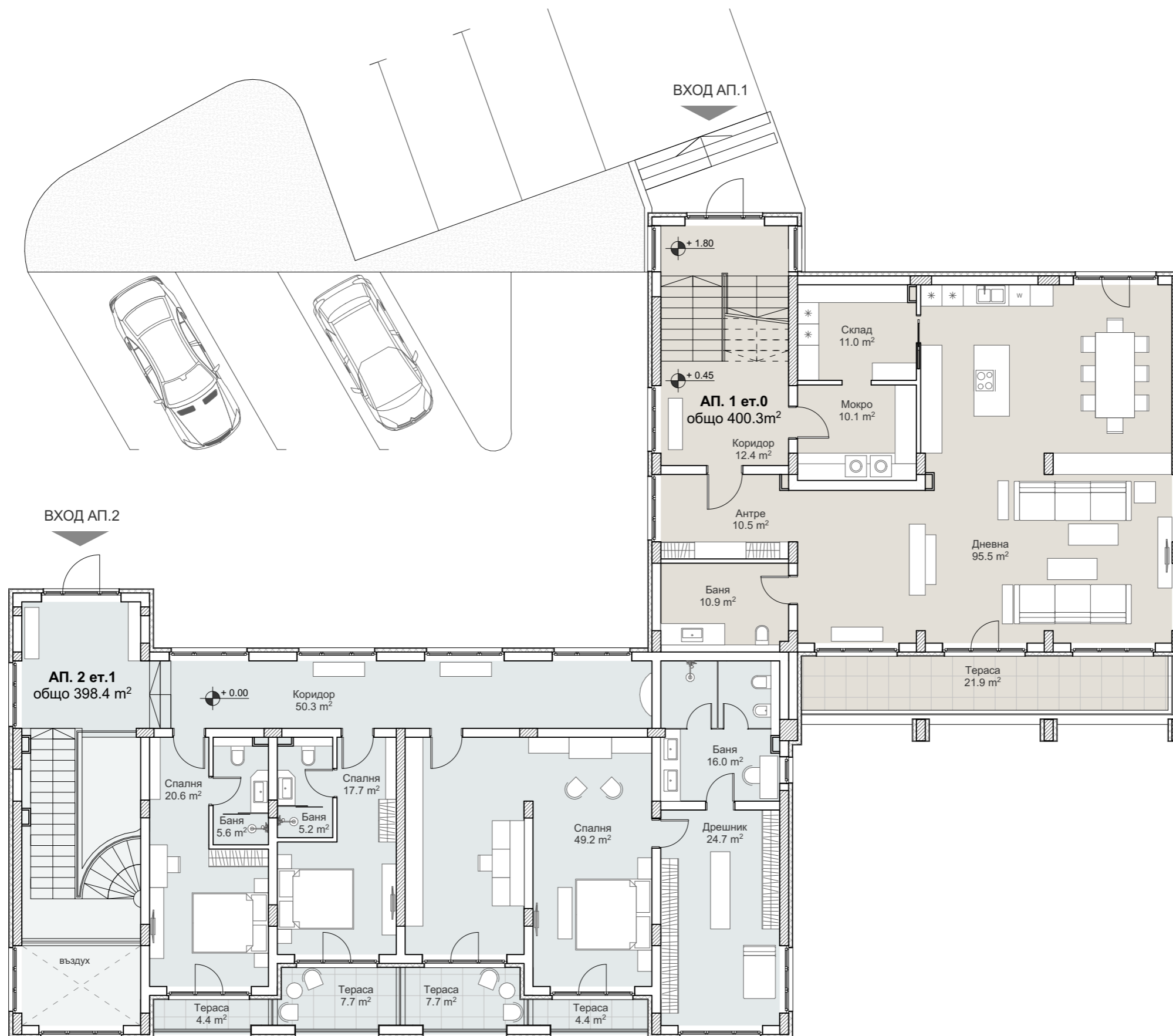
БЛОК 2 ПЛАН НА КОТА +0.00/+0.45
