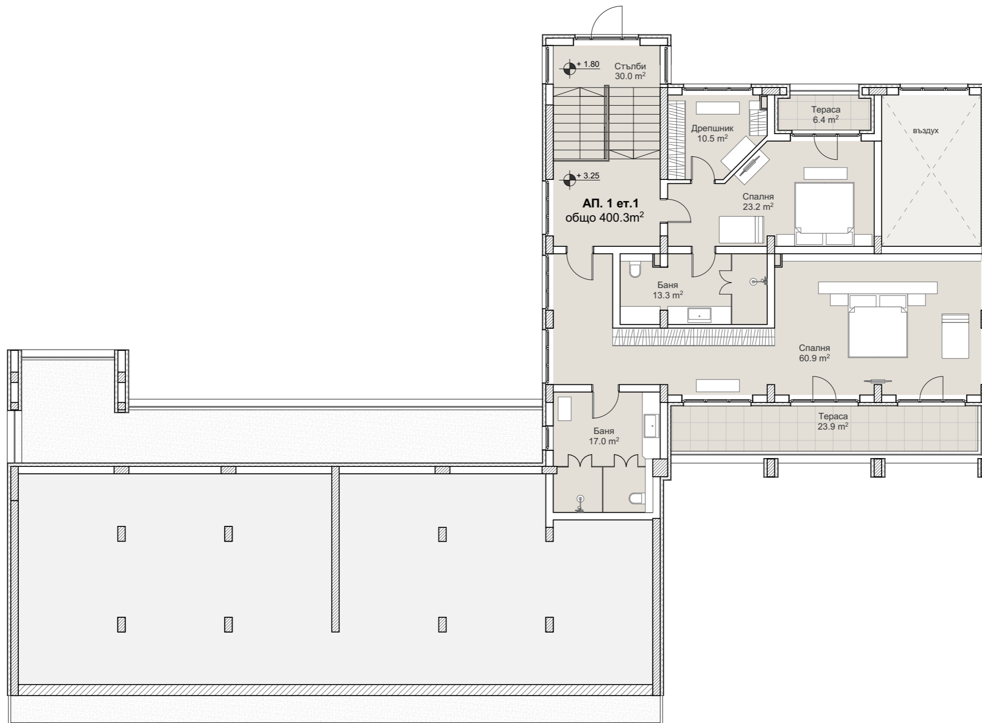
БЛОК 2 ПЛАН НА КОТА +3.25
