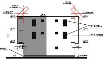
ФАСАДА ЮГОИСТОК М 1:100
