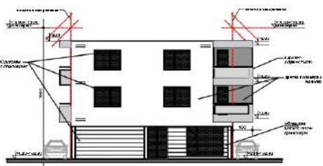
ФАСАДА СЕВЕРЗАПАД М 1:100
